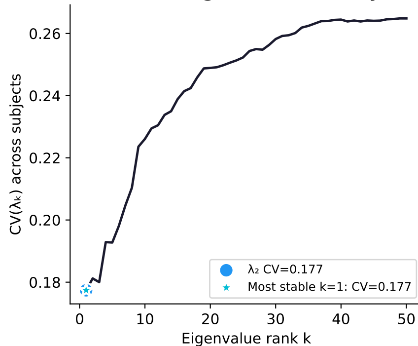
A. Raw Eigenvalue Stability
