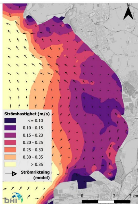
Figur 2-15 Maximal regional strömhastighet i Lommabukten. Pilarna visar medelriktningen för strömmen. Den lokalt genererade vågdrivna strömmen är exkluderad för att analysera enbart den regionala strömmen. Inom buktens grundare om (<4 m djup) dominerar den vågdrivna strömmen.
