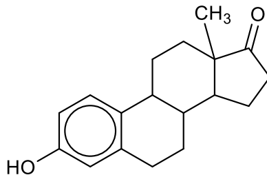
oestrone
