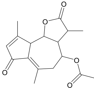
matricarin
