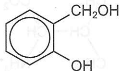
saligenin
