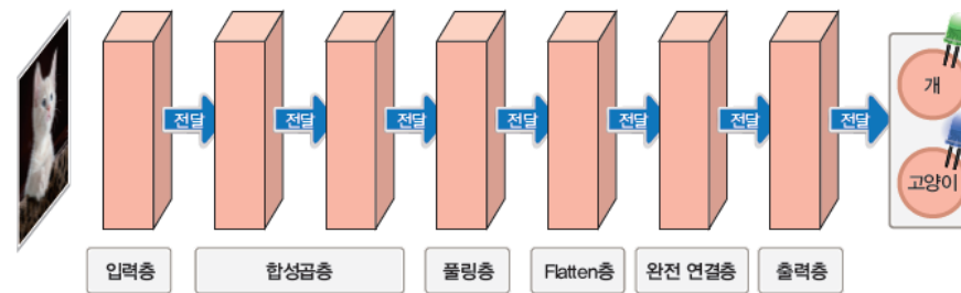
[그림 7-17] 합성곱 신경망의 예
