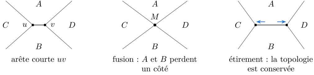
FIGURE 7 – Traitement d'une arête courte uv bordée par les cellules A et B .
