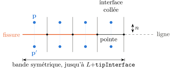
FIGURE 8 – Germes symétriques par rapport à la ligne de fissure : la médiatrice de \mathbf{p} et de son symétrique \mathbf{p}' est la ligne elle-même, qui est donc formée d'arêtes du pavage. La fissure est ouverte jusqu'à la pointe ; au-delà, la ligne se prolonge par une interface collée.
