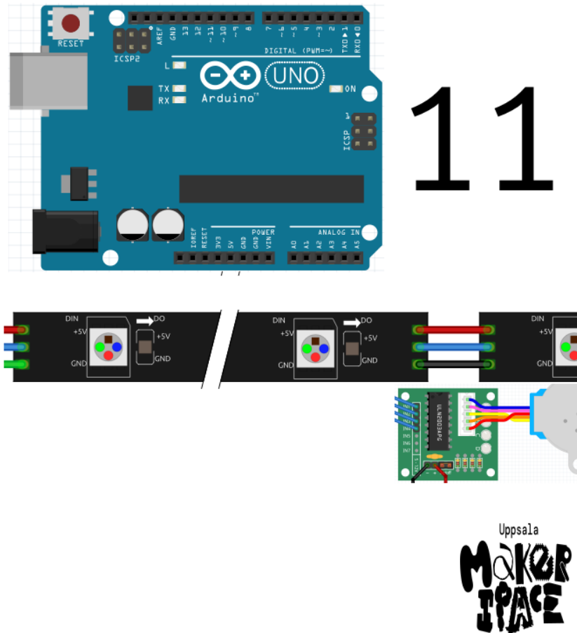
Figure 1: Bok 11: neopixlar och stegmotor
