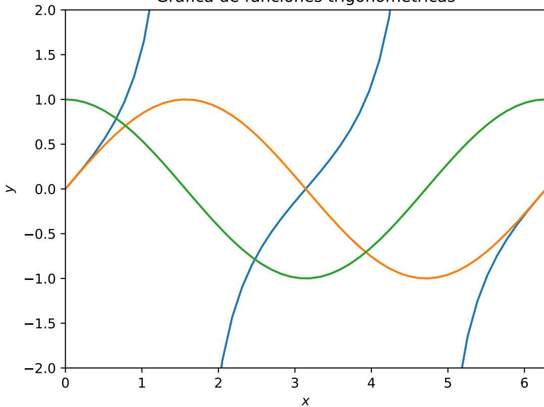
Gráfica de funciones trigonométricas
