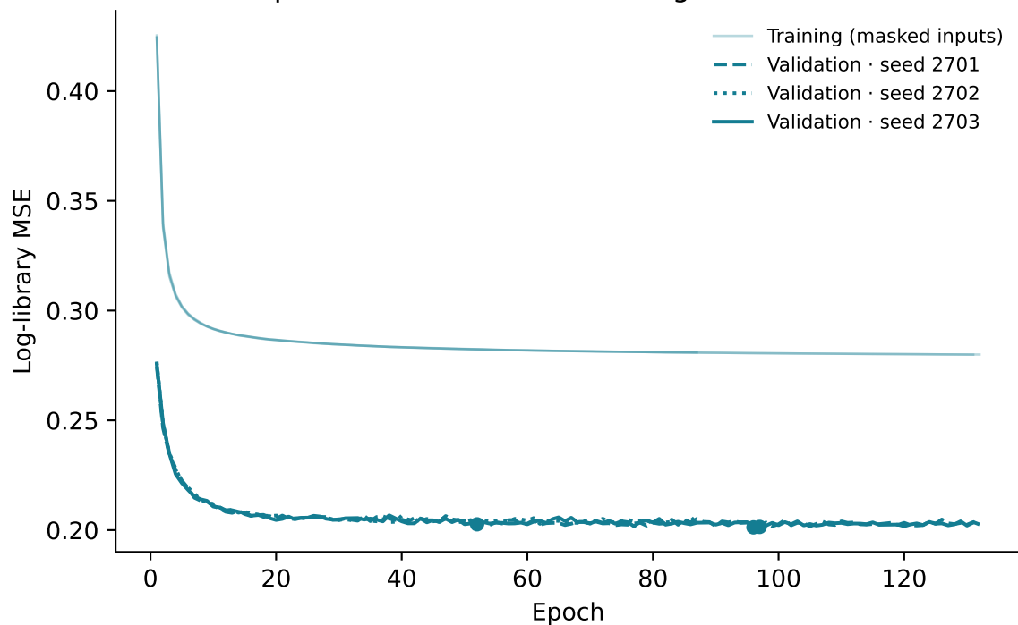
Fibroblast · denoising autoencoder
