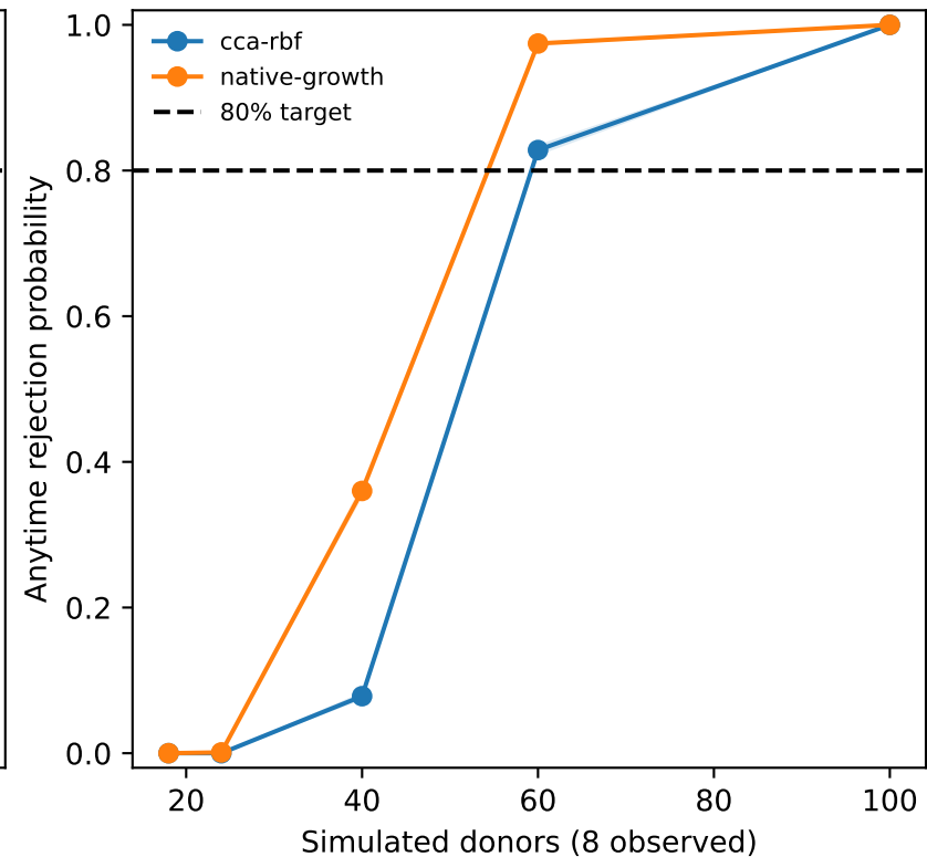
NB
