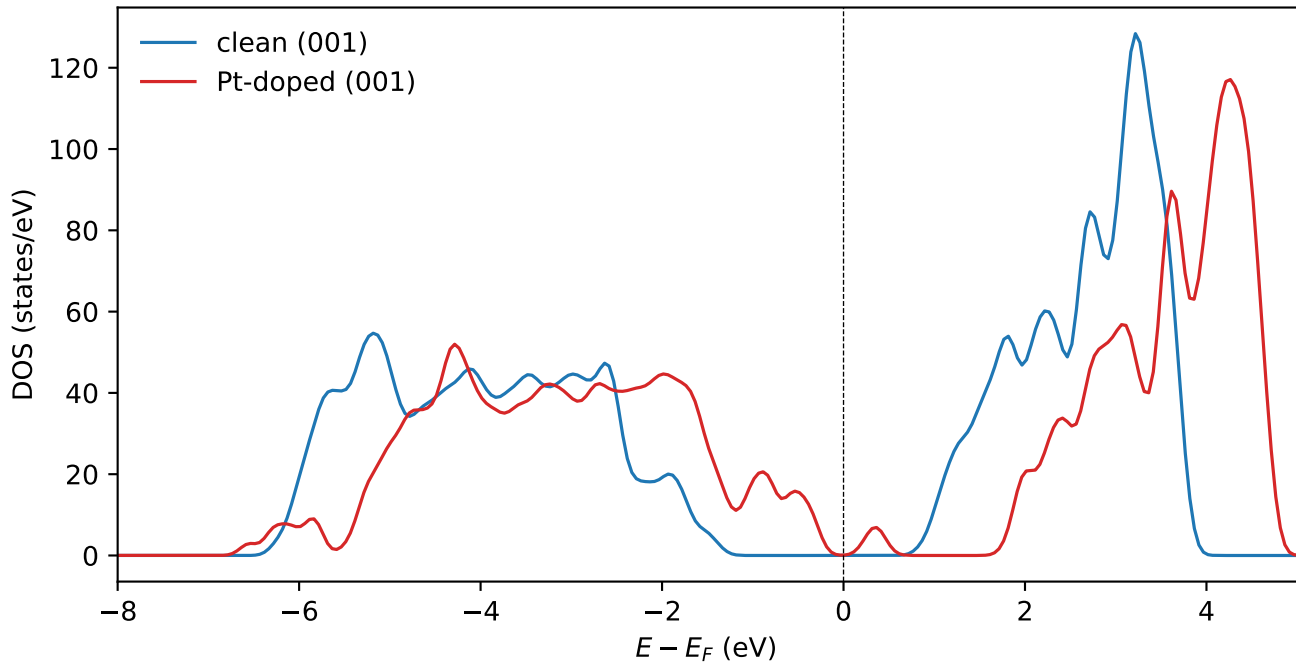
Total DOS: clean vs Pt-doped \text{La}_2\text{Ti}_2\text{O}_7(001)
