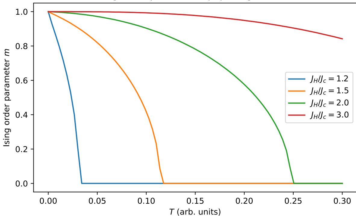
Ising order parameter (paper Fig. 3 inset)
