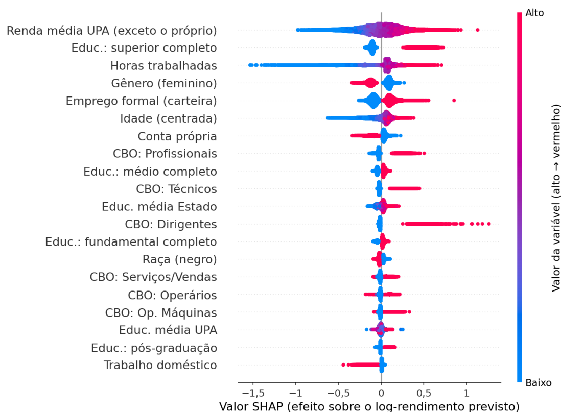
Figura 8. Contexto do bairro, diploma superior e jornada dominam a previsão de renda; a raça aparece na 14ª posição entre 28 preditores (SHAP, XGBoost, N_{\text{SHAP}} = 50.000 )
