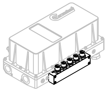
ISOMETRIC VIEW SCALE: 1 : 10
