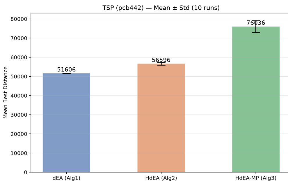
图 2: 柱状图: 三种算法均值和标准差对比 (误差线表示 \pm 1 标准差)
