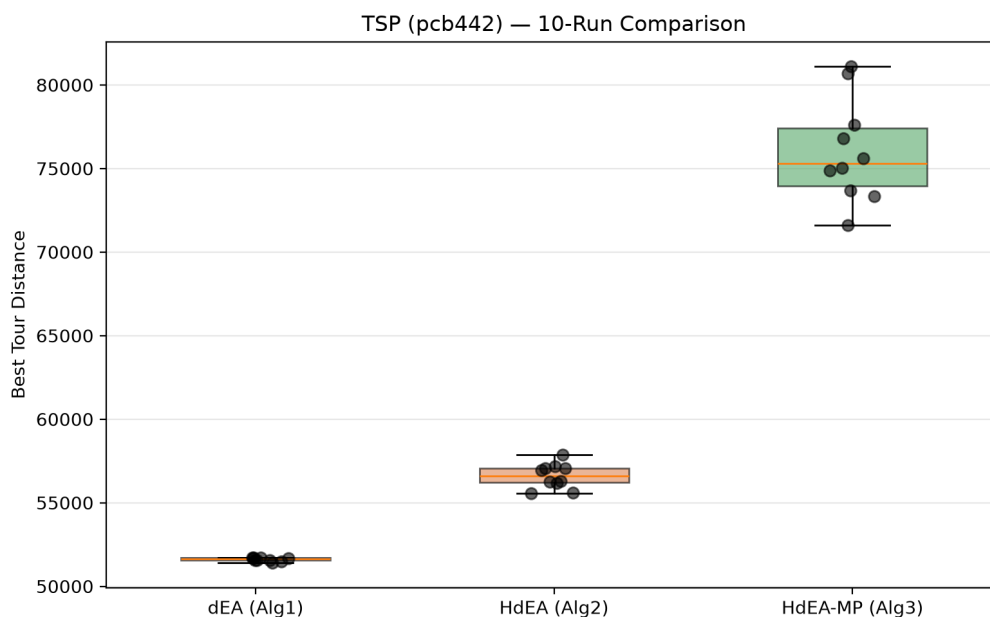
图 1: 箱线图: 三种算法 10 次运行结果分布
