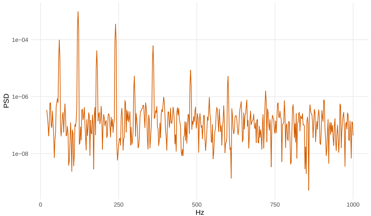
fig04 PSD (Hann, V 2 /Hz)
