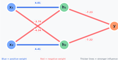
Input Layer
