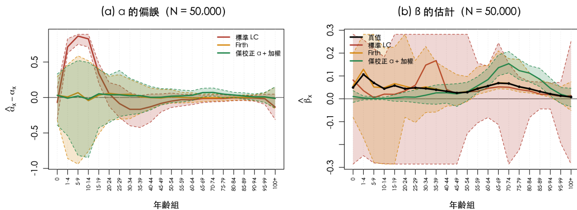
圖 11 標準 Lee-Carter、Firth 與僅校正 \alpha 加權的逐年齡分布 (人數五萬，5-95% 帶)
