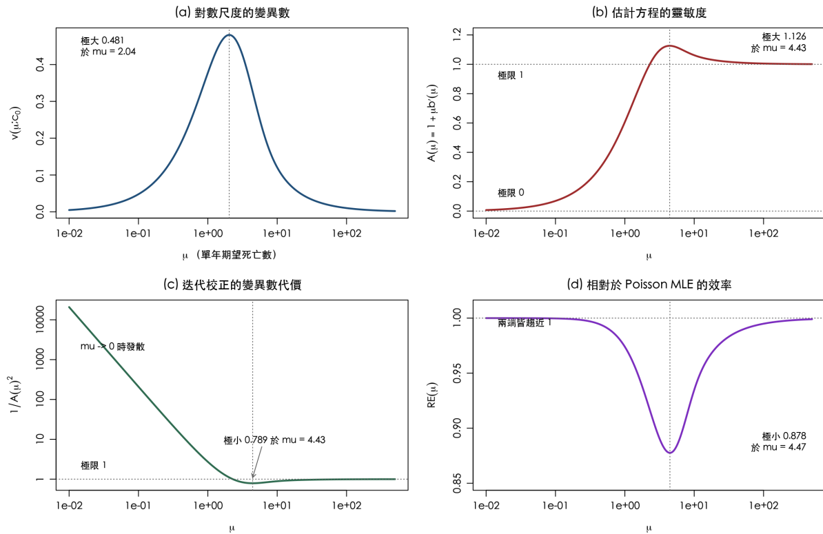
圖 2 四個二階解析量對期望死亡數的變化 ( c_0 = 0.5 ，橫軸取對數)。(a) 對數尺度的變異數 v(\mu; c_0) ，兩端趨於零而於 \mu = 2.04 取極大 0.481。(b) 估計方程的靈敏度 A(\mu) = 1 + \mu b'(\mu) ，兩端極限為 0 與 1，於 \mu = 4.43 取極大 1.126。(c) 迭代校正的變異數代價 1/A(\mu)^2 (縱軸亦取對數)， \mu \rightarrow 0 時發散，於 \mu = 4.43 取極小 0.789， \mu \rightarrow \infty 時趨於 1。(d) 相對於 Poisson 最大概似的效率，兩端皆趨近 1，於 \mu = 4.47 取極小 0.878。
