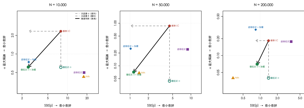
圖 10 \alpha 與 \beta 的取捨圖。由標準 Lee-Carter 出發，僅校正 \alpha 是垂直向下（只改善 \alpha ， \beta 完全不動）、逐格校正加權是水平向左（主要改善 \beta ），而僅校正 \alpha 加上加權則是對角線（兩者同時）。人數五萬時該點與 Firth 幾乎重合。
