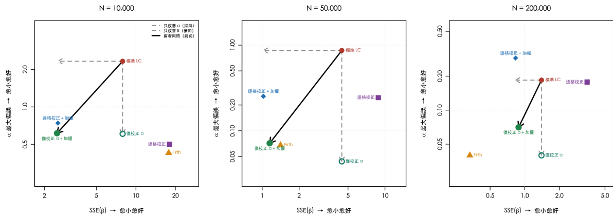
圖 10 \alpha 與 \beta 的取舍圖。由標準 LC 出發，僅校正 \alpha 是垂直向下（只改善 \alpha ， \beta 完全不動）、逐格校正加權是水平向左（主要改善 \beta ），而僅校正 \alpha 加上加權則是對角線（兩者同時）。人數五萬時該點與 Firth 幾乎重合。
