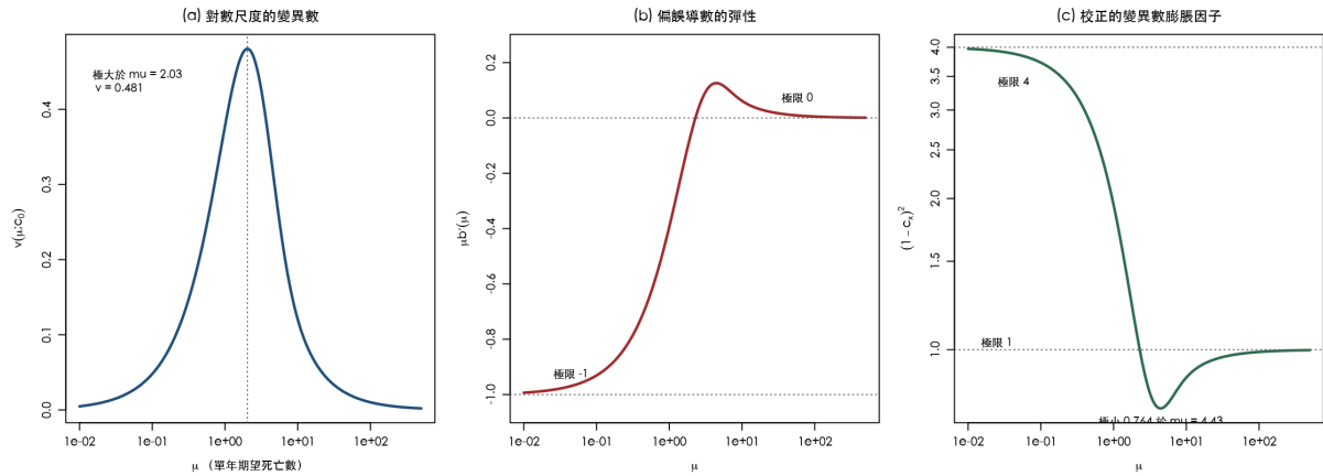
圖 2 三個二階解析量對期望死亡數的變化 ( c_0 = 0.5 , 橫軸取對數)。(a) 對數尺度的變異數 v(\mu; c_0) , 兩端趨於零而於 \mu = 2.03 取極大 0.481。(b) 偏誤導數的彈性 \mu b'(\mu) , 兩端極限為 -1 與 0 。(c) 校正的變異數膨脹因子 (1 - c_x)^2 (縱軸亦取對數), 由 4 遞減至極小 0.764 ( \mu = 4.43 ) 後回升至 1 。
