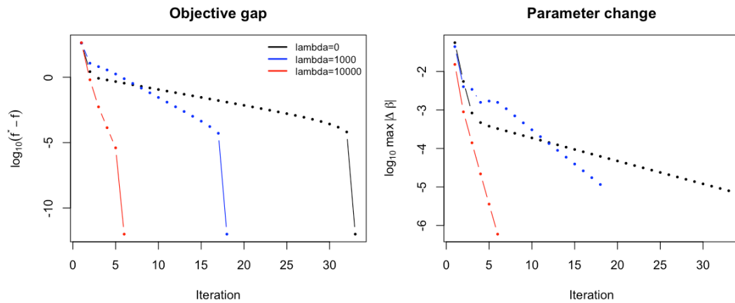
图 4 迭代收敛诊断。左：目标函数与最终值的间隙（对数尺度）；右：参数变动量。两者皆呈线性下降，即几何收敛。
