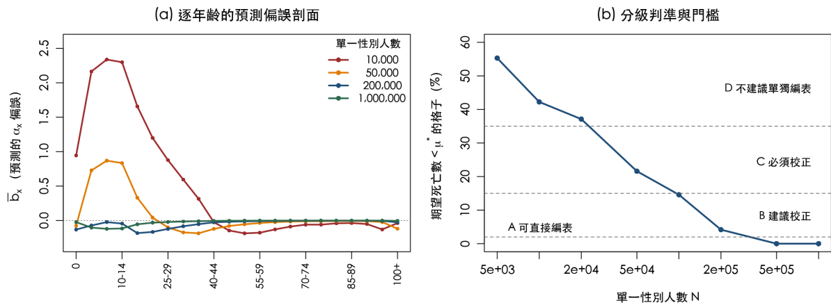
圖 4 事前可行性檢定的輸出
