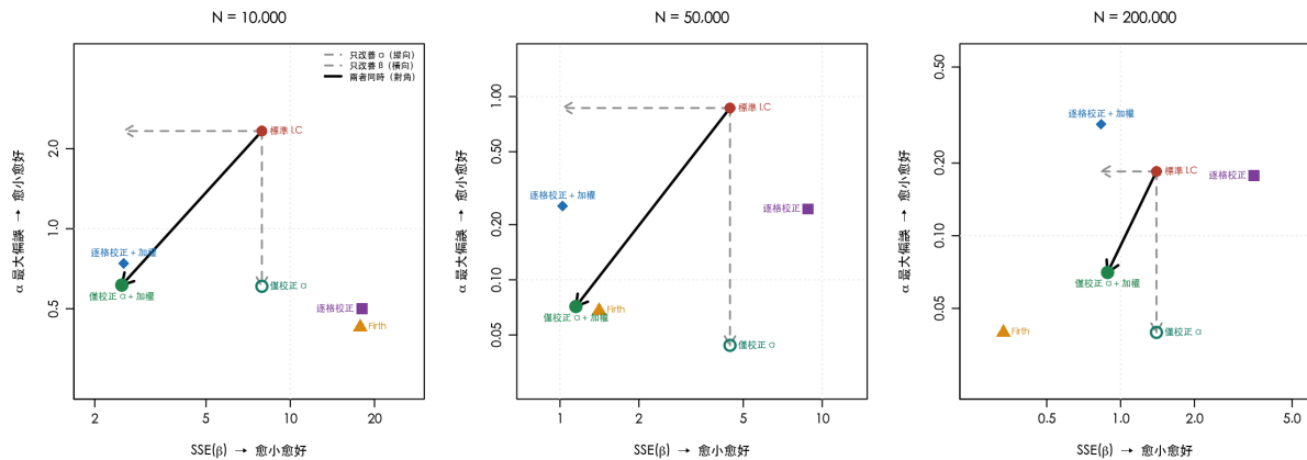
圖 10 \alpha 與 \beta 的取舍圖
