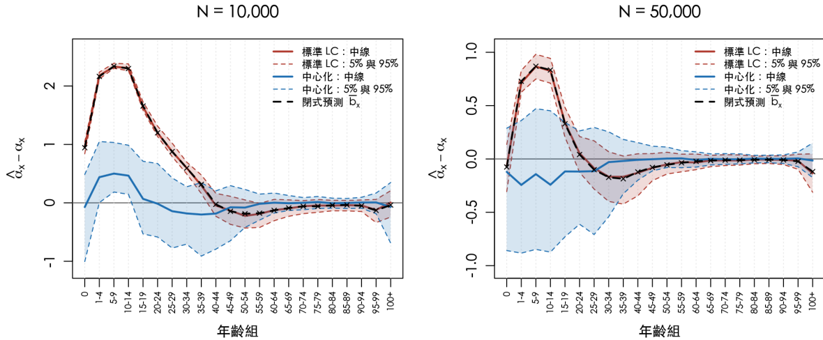
圖 3 \hat{\alpha}_x 的偏誤：5-95% 帶與閉式預測
