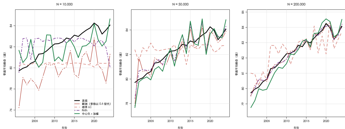
圖 9 零歲平均餘命的逐年序列（單次實現，亂數種子固定）
