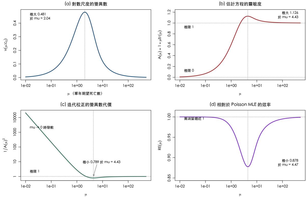
圖 2 四個二階解析量對期望死亡數的變化 ( c_0 = 0.5 , 橫軸取對數)
