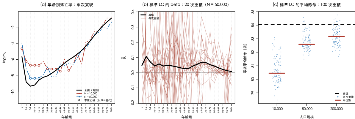
圖 1 小人口下 Lee-Carter 估計的震盪與偏誤（臺灣女性，以全國配適為真值）
