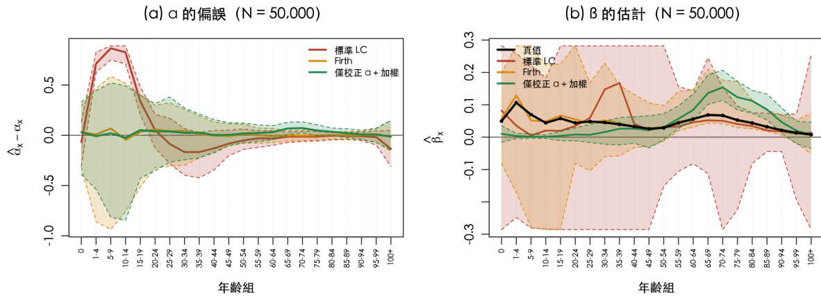
圖 11 標準 Lee-Carter、Firth 與僅校正 \alpha 加權的逐年齡分布（人數五萬，5-95% 帶） 註：(a) 逐年齡偏誤；(b) \hat{\beta}_x 的帶。
