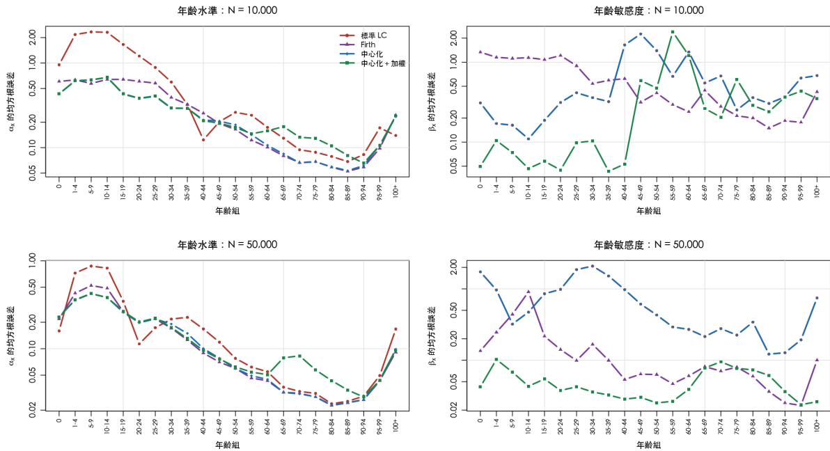
圖 8 逐年齡的均方根誤差 (縱軸取對數)
