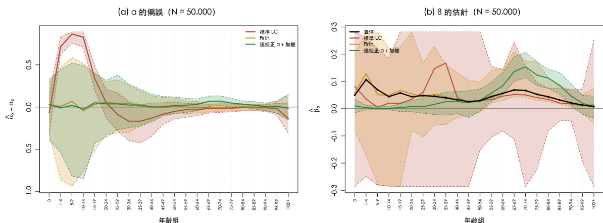
圖 7 標準 LC、Firth 與僅校正 \alpha 加權三者的逐年齡分布 ( N = 5 \times 10^4 , 5-95% 帶)。(a) 綠線在全年齡貼近零，標準 LC 則在幼年組隆起；(b) 綠色的帶最窄，其中線在多數年齡跟真值。
