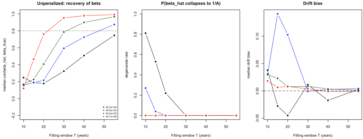
圖 3 配適期長度 T 與人口規模 N 的二因子結果。虛線為相關係數 0.8。
