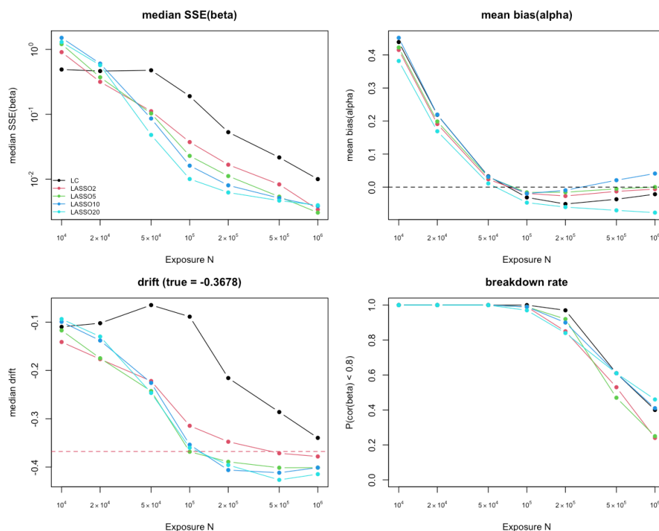
圖 2 暴露數與估計方法的蒙地卡羅模擬結果
