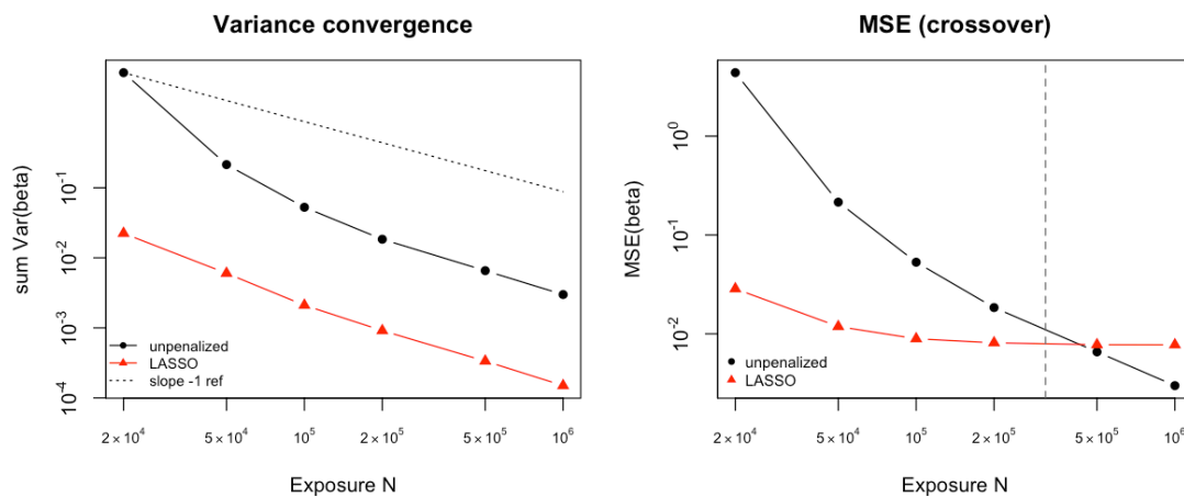
圖 7 變異數的收斂速度與 MSE 的交叉（重複 100 次）
