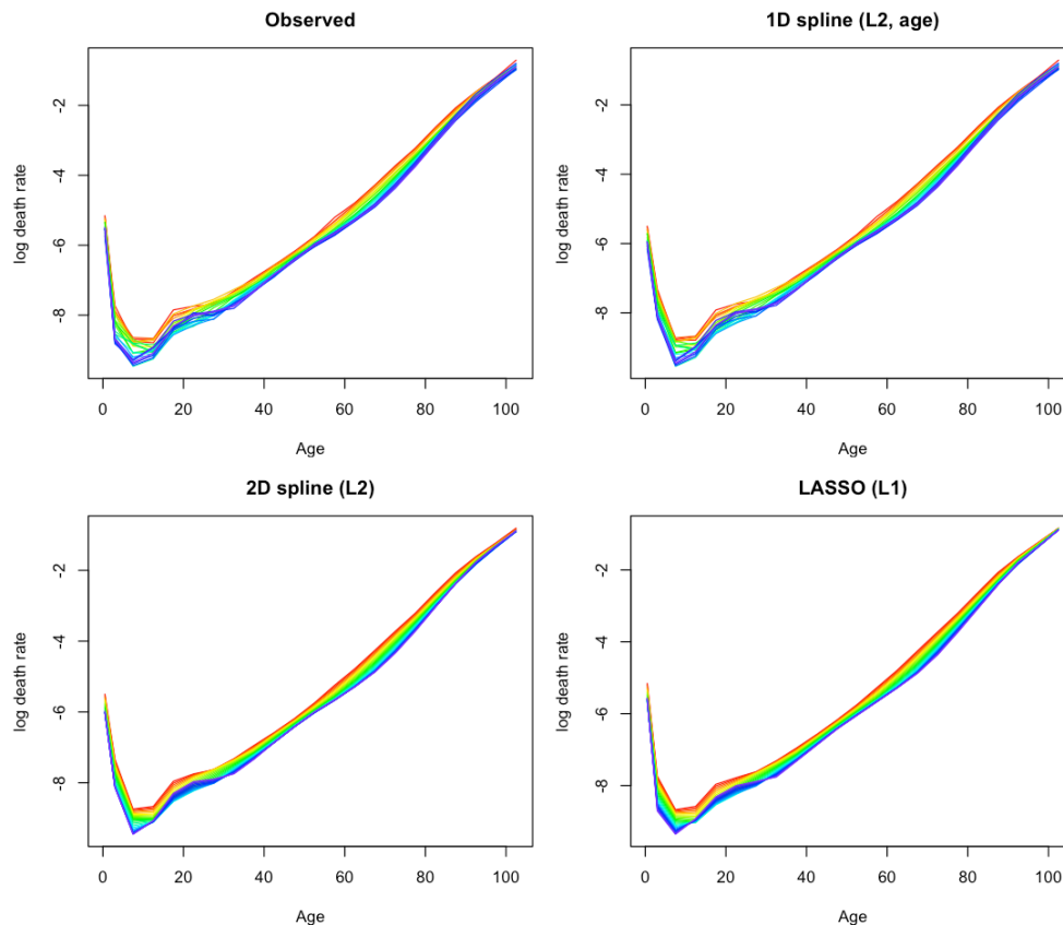
圖 1 三種修勻法的死亡率曲面（女性 2001~2024 年，每條線為一年）
