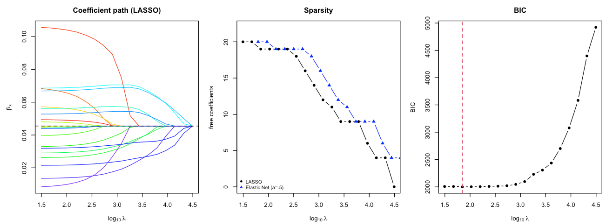
圖 5 LASSO 的係數路徑、稀疏度與 BIC（女性 2001~2024 年）
