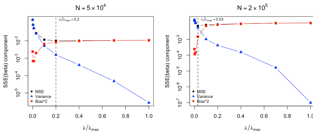
圖 6 偏誤—變異數權衡（LASSO，重複 100 次）；虛線為 MSE 的最小值位置
