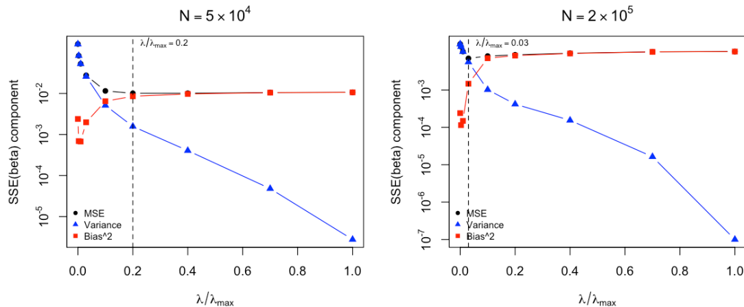
圖 6 偏誤—變異數權衡（LASSO，重複 100 次）；虛線為 MSE 的最小值位置
