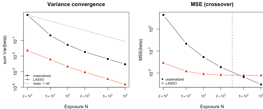
圖 7 變異數的收斂速度與 MSE 的交叉（重複 100 次）
