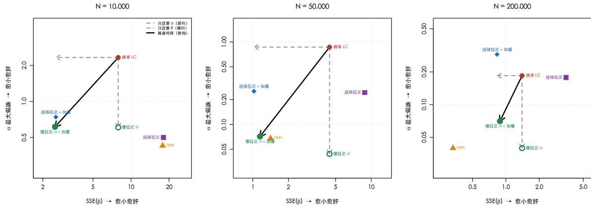
圖 10 \alpha 與 \beta 的取舍圖。由標準 LC 出發，僅校正 \alpha 是垂直向下（只改善 \alpha ， \beta 完全不動）、逐格校正加權是水平向左（主要改善 \beta ），而僅校正 \alpha 加上加權則是對角線（兩者同時）。 N = 5 \times 10^4 時該點與 Firth 幾乎重合。
