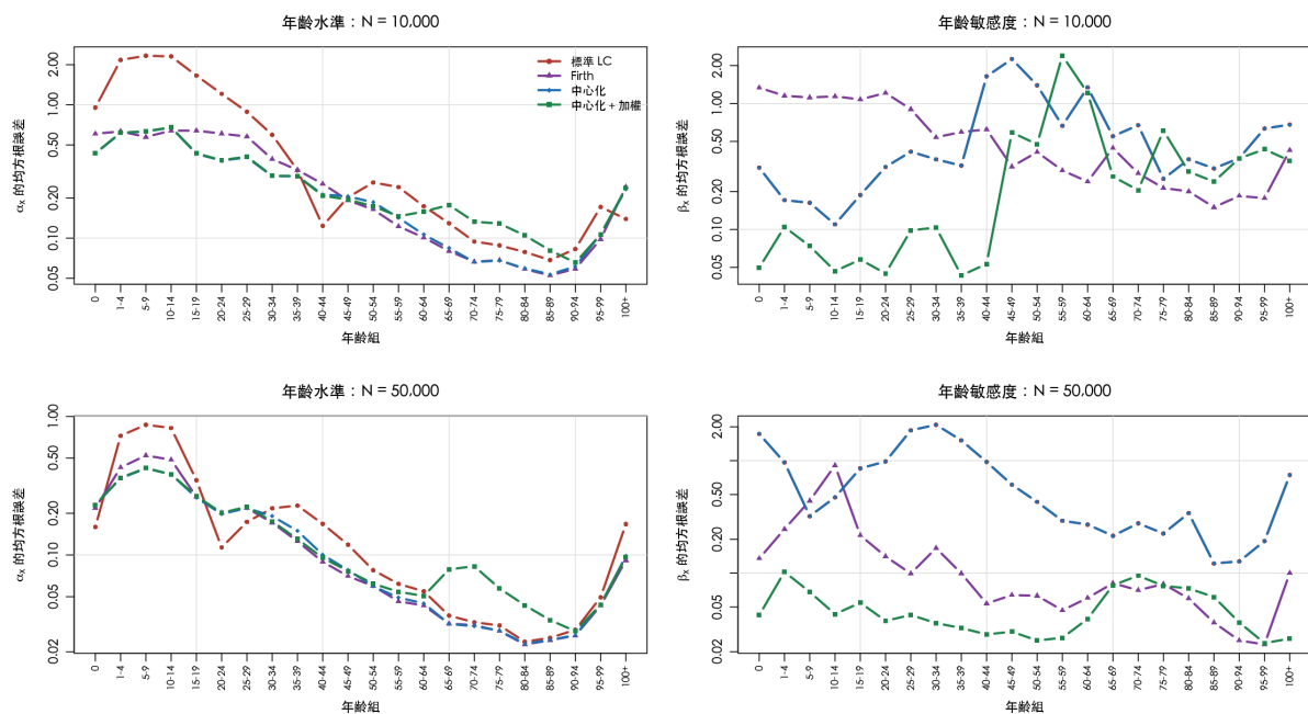
圖 8 逐年齡的均方根誤差（縱軸取對數）。上列為 N = 10^4 、下列為 N = 5 \times 10^4 ；左欄為年齡水準 \alpha_x 、右欄為年齡敏感度 \beta_x 。 \alpha 的改善集中在左側死亡數少的年齡， \beta 的改善則遍及全部年齡。右欄中標準 LC（紅）的線完全被「中心化」（藍）覆蓋，因為僅校正 \alpha_x 不改變中心化矩陣，兩者的 \hat{\beta}_x 逐位相同。
