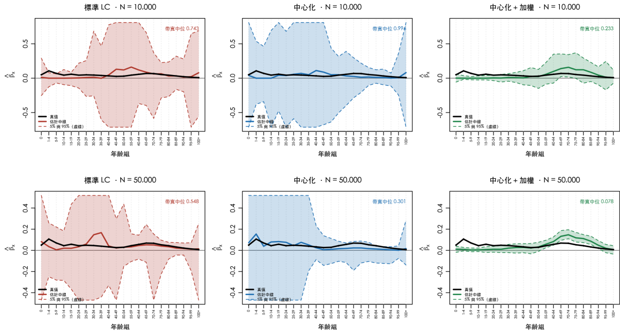
圖 5 \hat{\beta}_x 的 5–95% 帶 (每格一個估計量, 上列 N = 10^4 、下列 N = 5 \times 10^4 )。黑線為真值。與圖 3 的 \alpha 相反, \beta 的帶很寬而中線大致罩住真值, 是變異數主導的樣子。中心化單獨反而使帶變寬 (0.743 \rightarrow 0.996), 須加上資訊加權才收窄 ( \rightarrow 0.233)。
