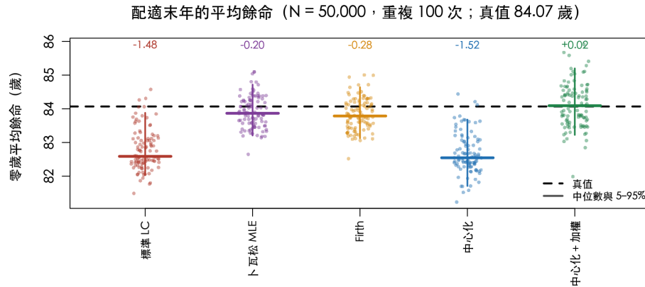
圖 7 配適末年零歲平均餘命的 100 次重複 ( N = 5 \times 10^4 )。虛線為真值 84.07 歲，各估計量上方標示其中位偏誤。標準 LC 低估 1.48 歲，中心化加權則為 +0.02 歲。
