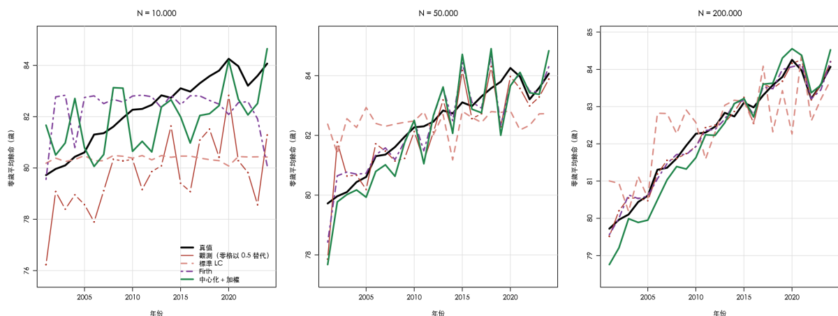
圖 9 零歲平均餘命的逐年序列（單次實現，亂數種子固定）。觀測序列（深紅）在人數一萬時上下跳動逾兩歲，而真值（黑）平滑遞增；標準 LC（淺紅虛線）雖把跳動壓下，卻同時把整條趨勢壓平，其全距僅為真值的六成四。人數二十萬時三條配適線已大致與真值重合。
