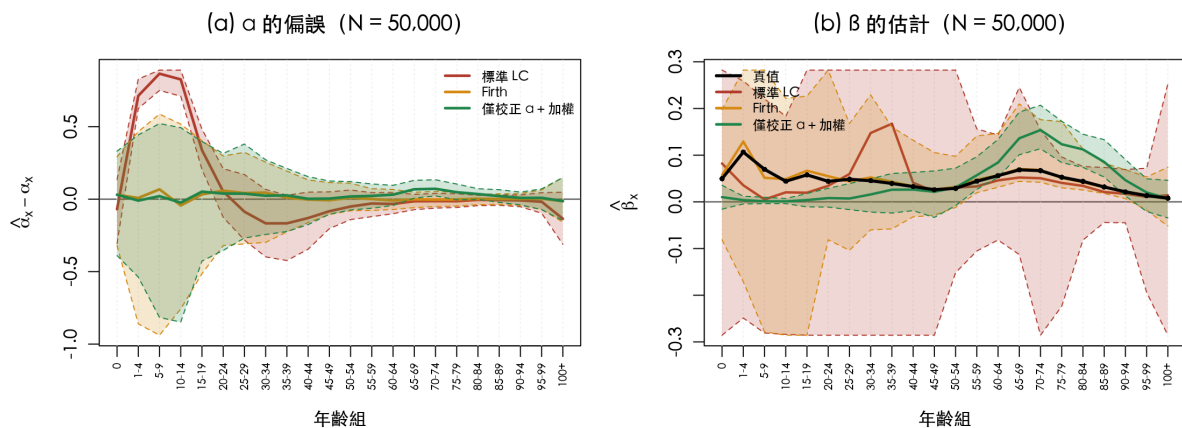
圖 11 標準 LC、Firth 與僅校正 \alpha 加權三者的逐年齡分布（ N = 5 \times 10^4 ，5–95% 帶）。(a) 綠線在全年齡貼近零，標準 LC 則在幼年組隆起；(b) 綠色的帶最窄，其中線在多數年齡跟上真值。
