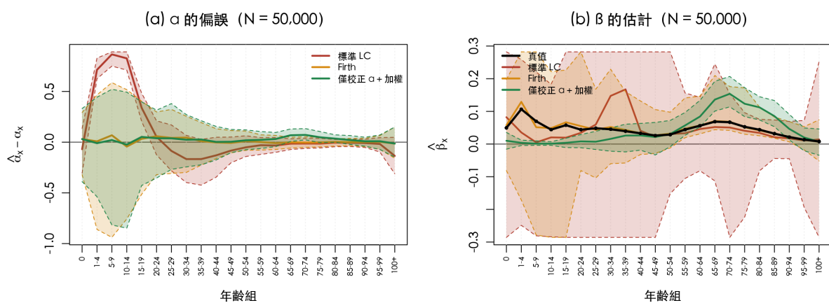
圖 9 標準 LC、Firth 與僅校正 \alpha 加權三者的逐年齡分布 ( N = 5 \times 10^4 , 5-95% 帶)。(a) 綠線在全年齡貼近零，標準 LC 則在幼年組隆起；(b) 綠色的帶最窄，其中線在多數年齡跟上真值。
