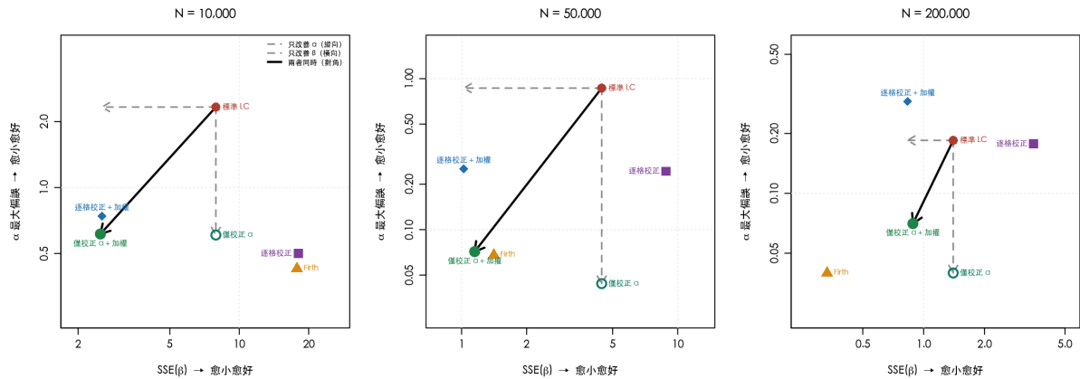
圖 8 \alpha 與 \beta 的取舍圖。由標準 LC 出發，僅校正 \alpha 是垂直向下（只改善 \alpha ， \beta 完全不動）、逐格校正加權是水平向左（主要改善 \beta ），而僅校正 \alpha 加上加權則是對角線（兩者同時）。 N = 5 \times 10^4 時該點與 Firth 幾乎重合。
