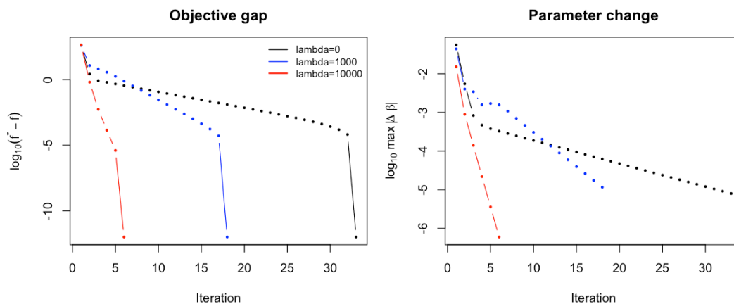
圖 4 迭代收斂診斷。左: 目標函數與最終值的間隙 (對數尺度); 右: 參數變動量。兩者皆呈線性下降, 即幾何收斂。
