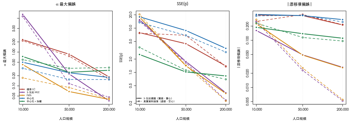
圖 6 三項指標隨人口規模的變化（縱軸取對數）
