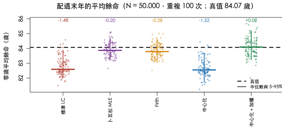
圖 7 配適末年零歲平均餘命的 100 次重複（人數五萬）
