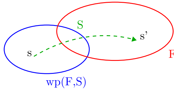
Figura 9: s è lo stato in cui è vera wp(F, S) e s' è lo stato in cui è vera F . S è un insieme di statements o istruzioni e F è una formula della logica del primo ordine.
