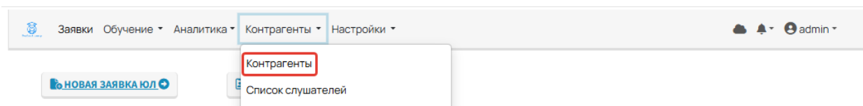
Рис.1. Раздел «Контрагенты»
