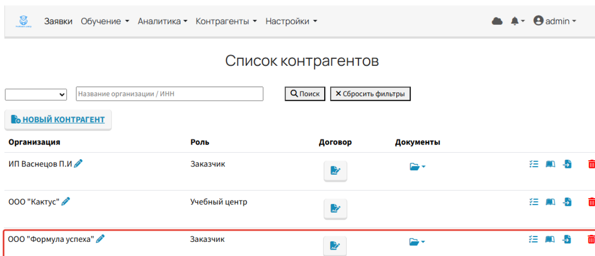
Рис.5. Список контрагентов
