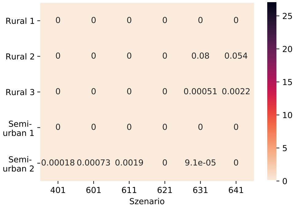
Leitungsüberlastung [%]
