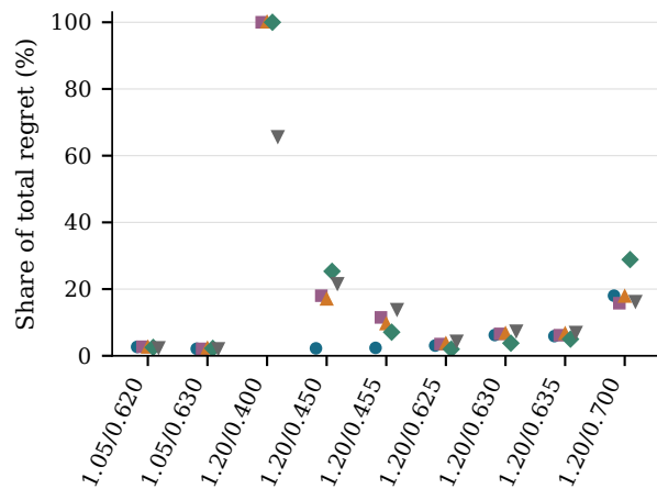
(d) Loss share of worst 1%
