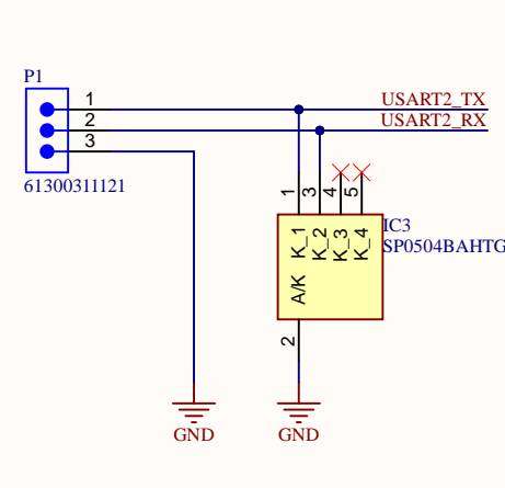
UART
