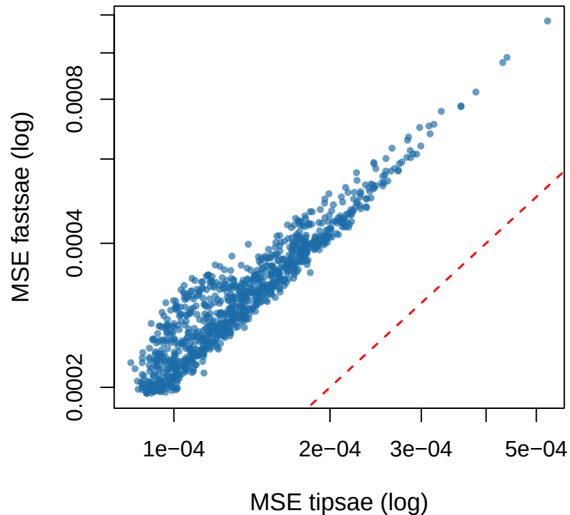
(b) MSE
