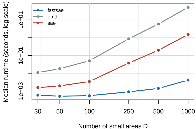
(c) Spatio-temporal Fay–Herriot
