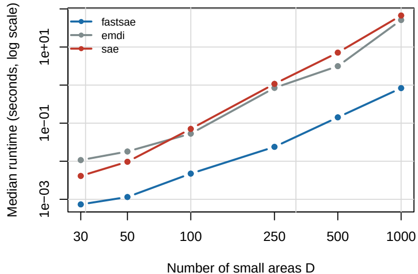
(d) Hierarchical Bayes Gaussian
