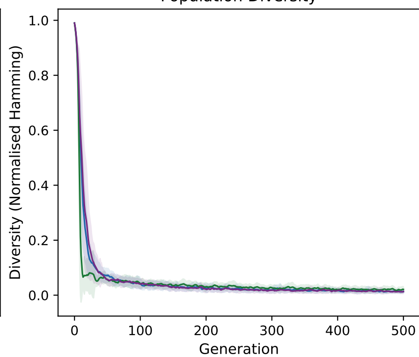
Population Diversity
