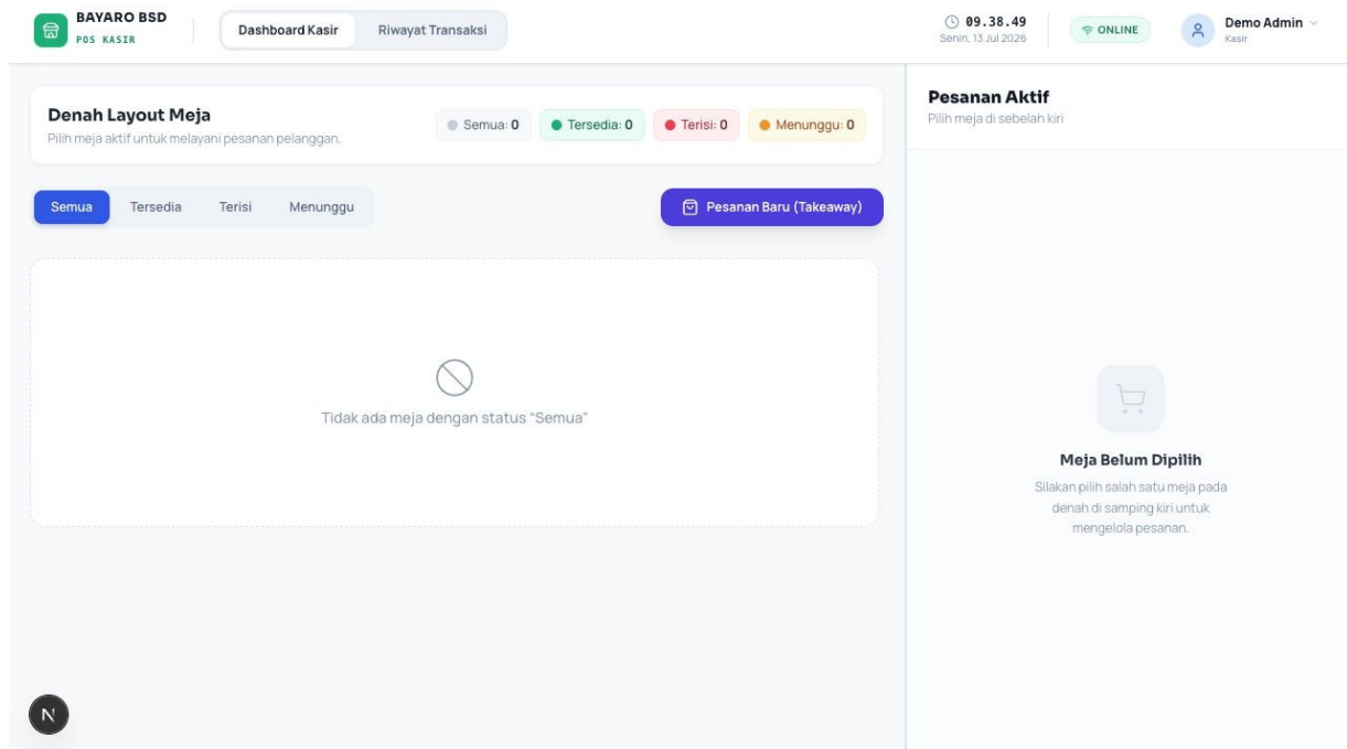
Gambar 6. POS Kasir: status meja, filter meja, pesanan takeaway, dan panel pesanan aktif.
