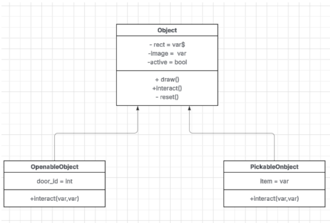
Figure 10: Diagramme de classe 3
