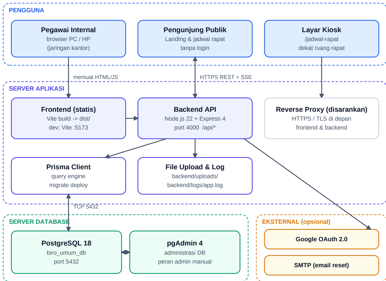
Gambar 1. Topologi infrastruktur
