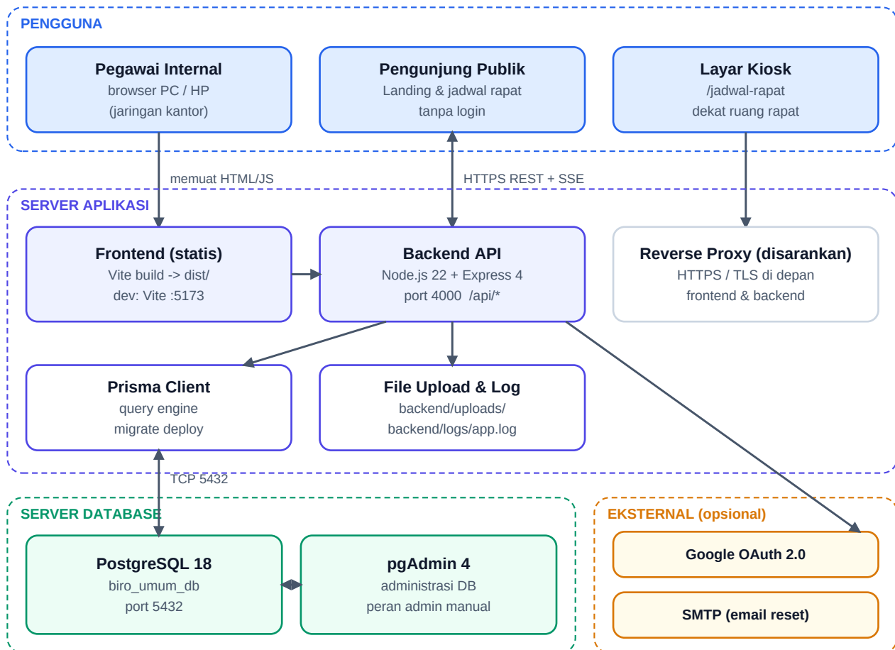
Gambar 1. Topologi infrastruktur
