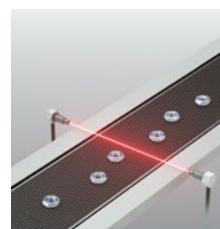
透過型は設置が面倒
