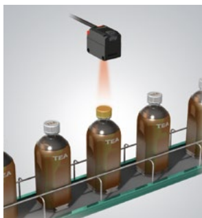
キャップの品種判別
