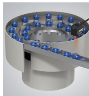
パーツフィーダー上の 部品転倒確認
