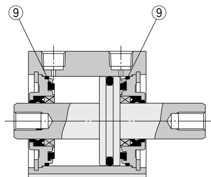
ワンタッチ管継手付
