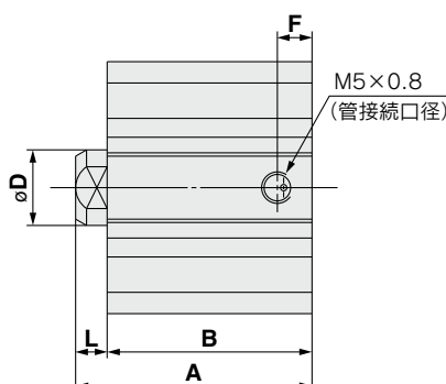
押出し形
