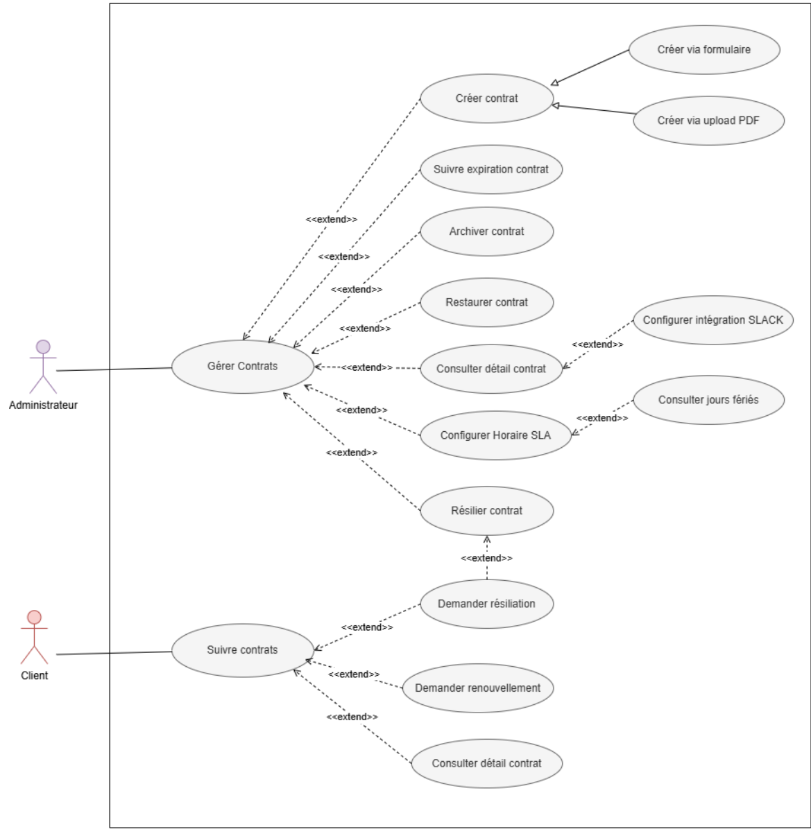
FIGURE IV.2 – Diagramme des cas d'utilisation « Gérer Contrats »
