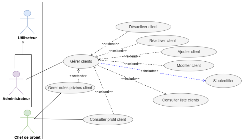
FIGURE IV.3 – Raffinement de cas d'utilisation « Gérer clients »
