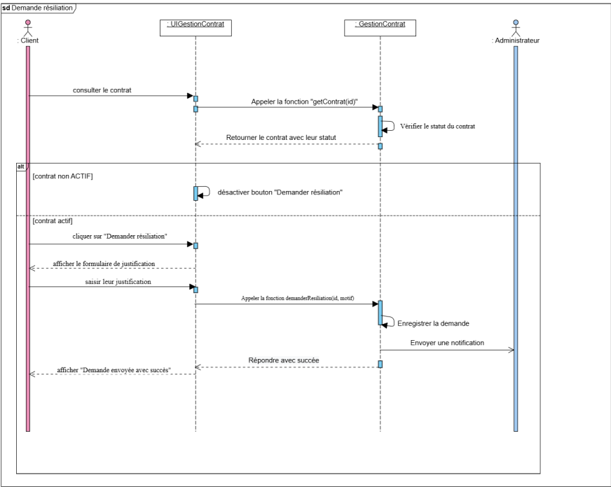
FIGURE IV.4 – Diagramme de séquence du cas d'utilisation « Demande Résiliation »
