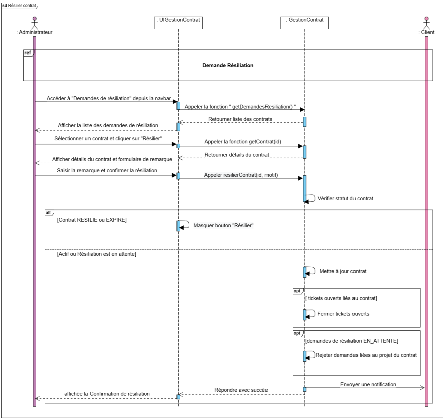
FIGURE IV.5 – Diagramme de séquence du cas d'utilisation « Résilier contrat »
