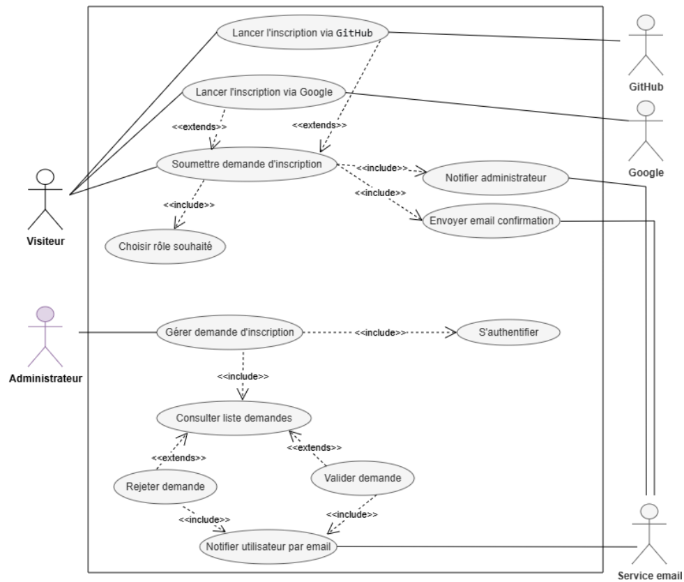
FIGURE III.2 – Raffinement de cas d'utilisation « Demander accès via OAuth »
