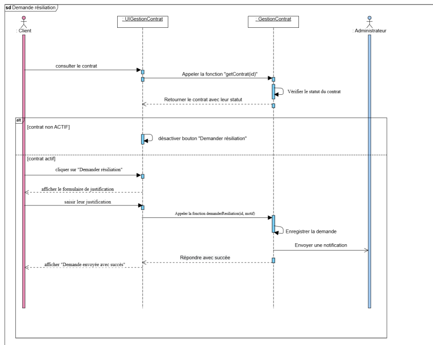
FIGURE IV.3 – Diagramme de séquence du cas d'utilisation « Demande Résiliation »
