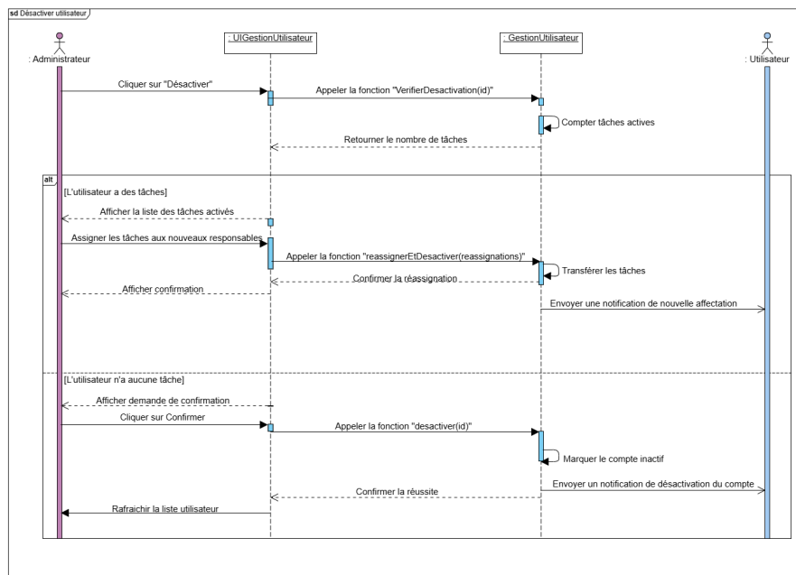
FIGURE III.10 – Diagramme de séquence du cas d'utilisation « Désactiver utilisateur »
