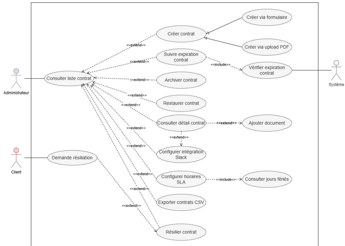
FIGURE IV.2 – Diagramme des cas d'utilisation « Gérer Contrats »
