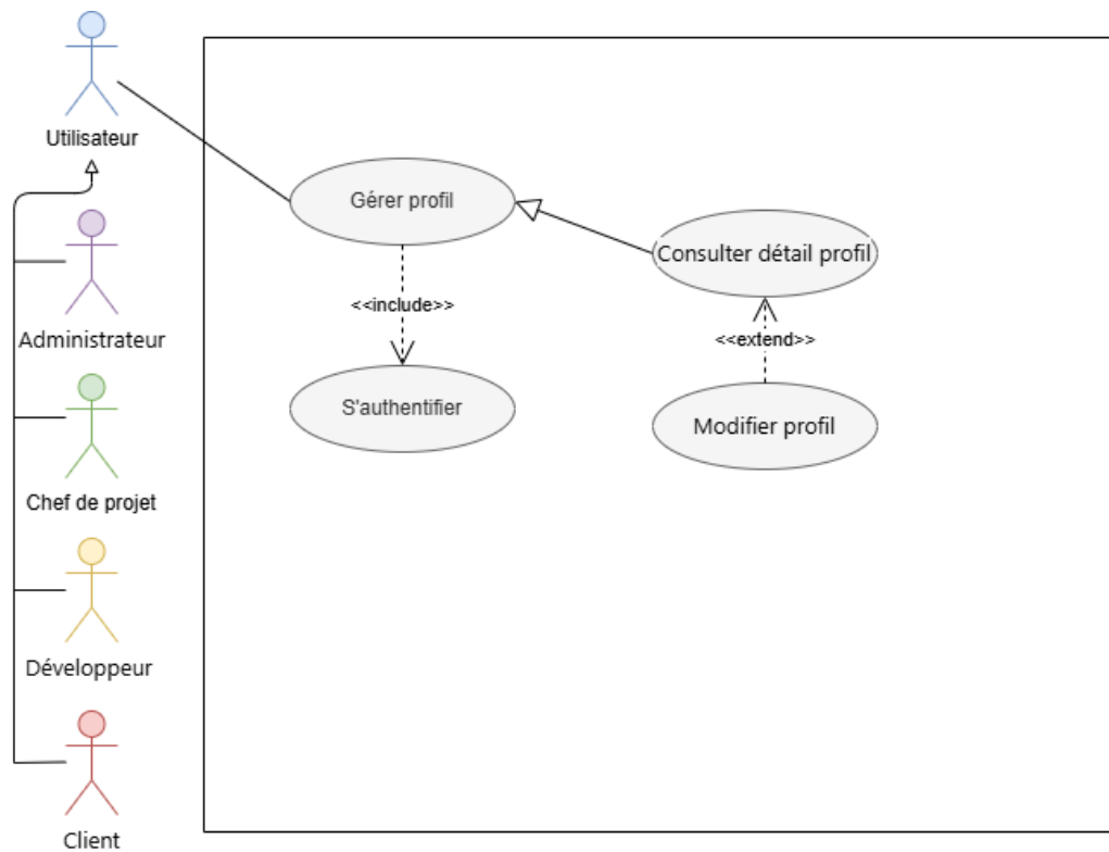
FIGURE III.4 – Raffinement de cas d'utilisation « Gérer Profil »
