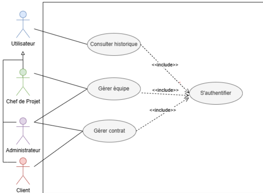
FIGURE IV.1 – Diagramme des cas d'utilisation du deuxième sprint
