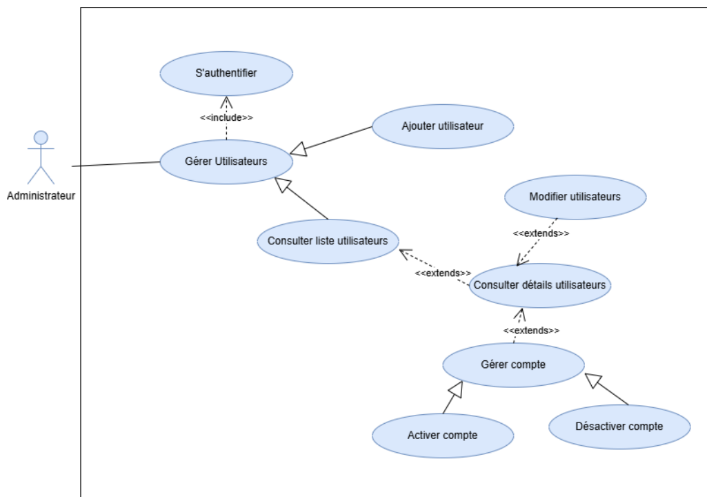
FIGURE IV.2 – Diagramme des cas d'utilisation « Gérer utilisateurs »
