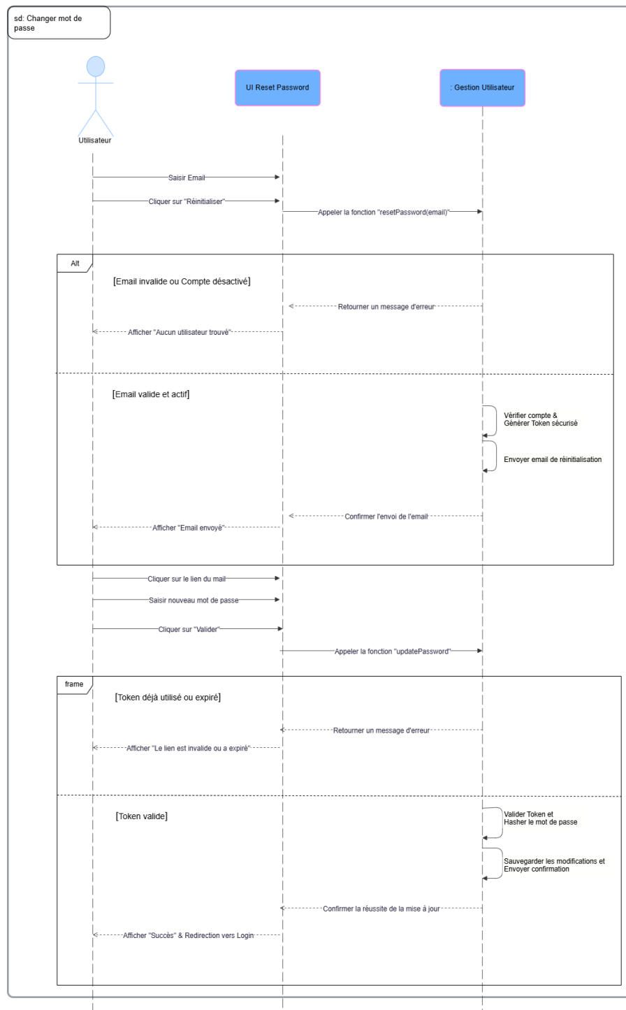
FIGURE III.7 – Diagramme de séquence du cas d'utilisation « Mot de passe oublié »
