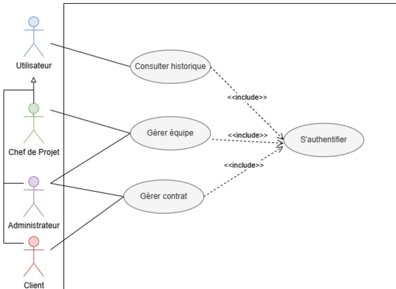
FIGURE IV.1 – Diagramme des cas d'utilisation du deuxième sprint
