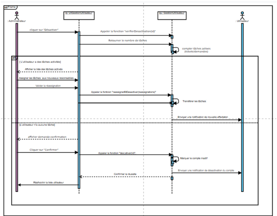
FIGURE III.10 – Diagramme de séquence du cas d'utilisation « Désactiver utilisateur »
