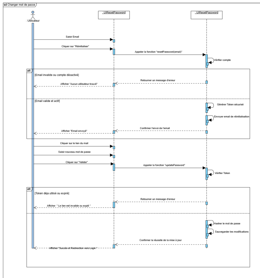
FIGURE III.9 – Diagramme de séquence du cas d'utilisation « Mot de passe oublié »
