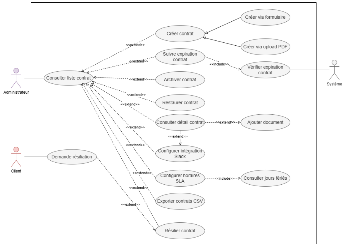
FIGURE IV.2 – Diagramme des cas d'utilisation « Gérer Contrats »
