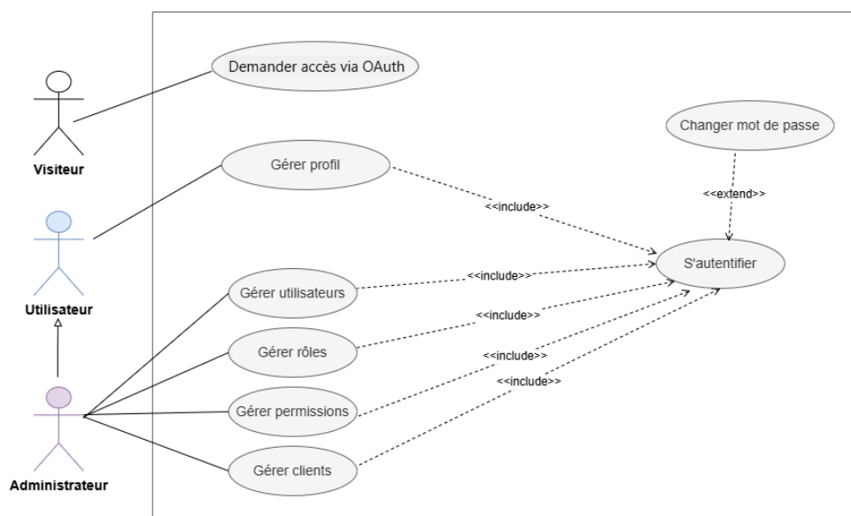
FIGURE III.1 – Diagramme des cas d'utilisation du premier sprint
