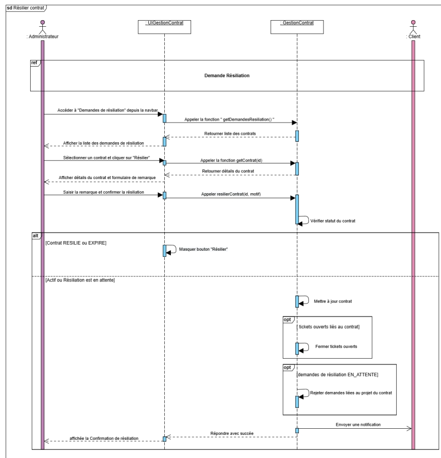
FIGURE IV.3 – Diagramme de séquence du cas d'utilisation « Résilier contrat »
