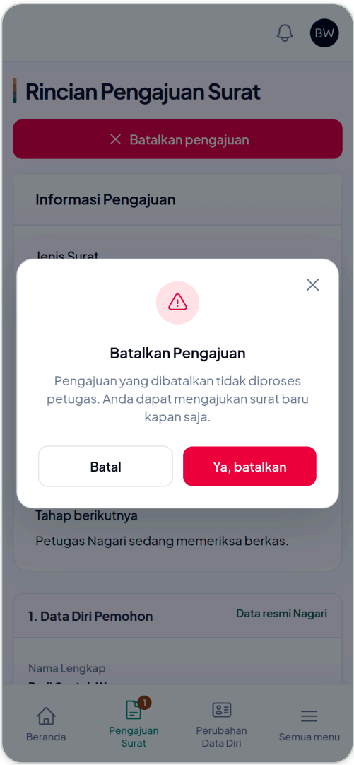
Gambar 3.15 — Konfirmasi pembatalan
